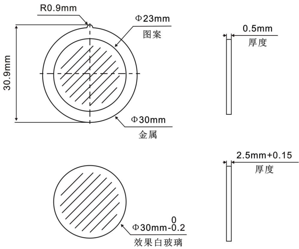
旋转图案片尺寸图：
