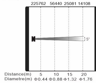
Min. Spot Mode Intensity LUX (5°)
