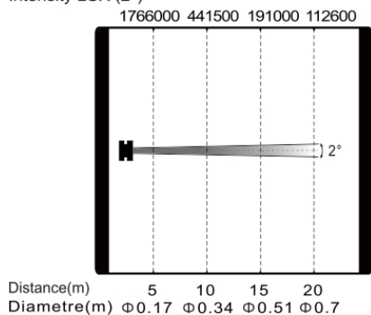
Min. Beam Mode Intensity LUX (2°)
