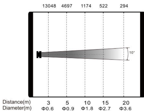
Intensity LUX(10°)
