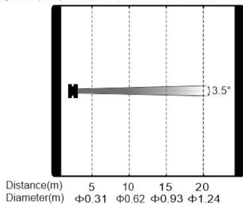
(SL750PH Pro) Min. Beam angle
