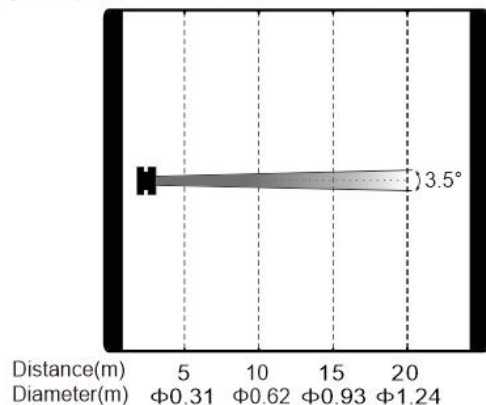
(SL750PH Pro) Min. Beam angle
