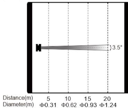
SL880PH IP Pro Intensity LUX (3.5°) 68799 17200 7664 4300
